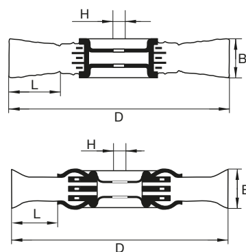
Afmetingen ronde borstels
