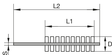
Afmetingen buisborstel
