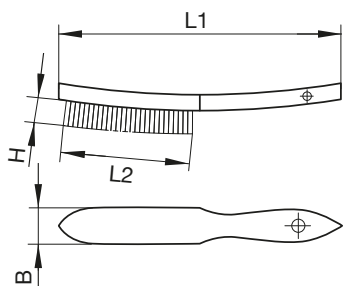
Afmetingen handborstels
