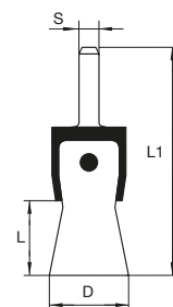
Afmetingen penseelborstels
